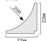
寸法図
